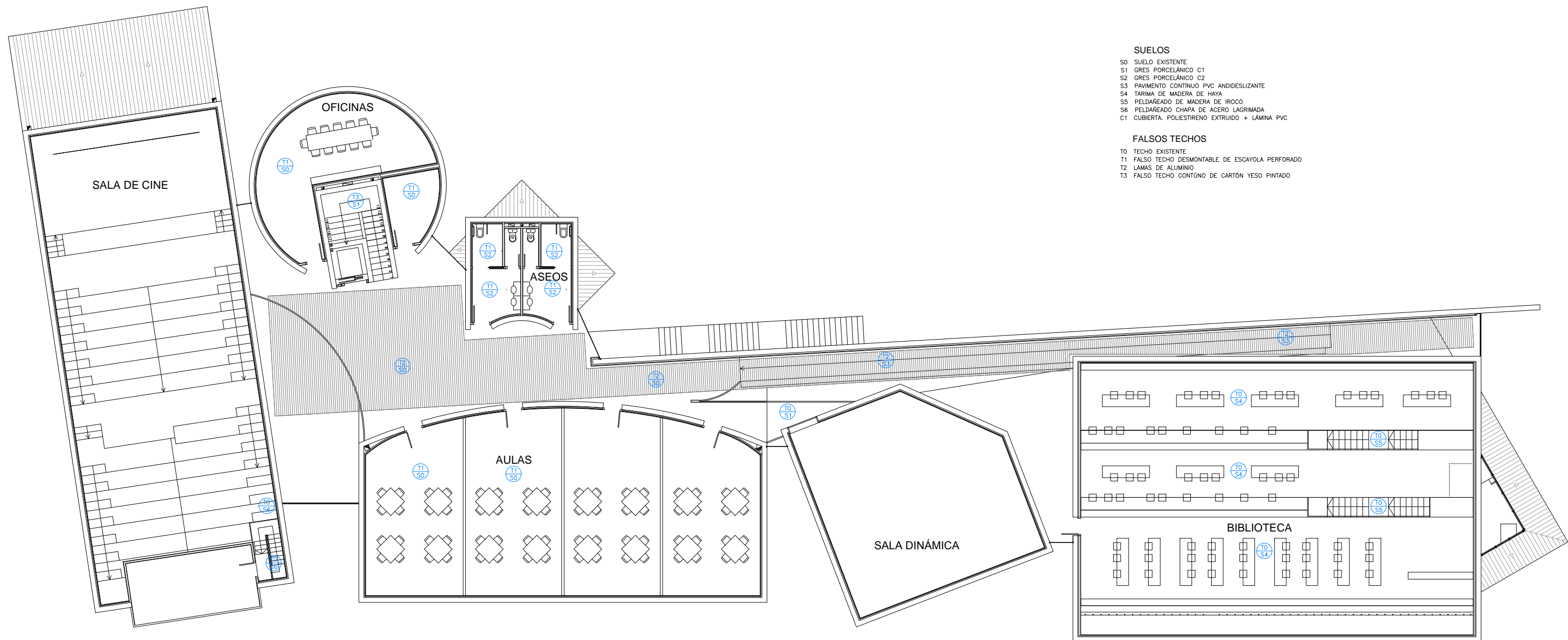
PLANTA PRIMERA
