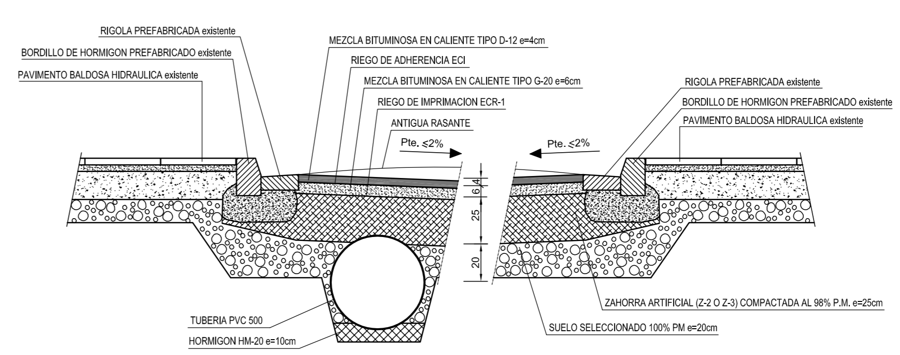
DETALLE CONSTRUCTIVO ESCALA: 1/20
